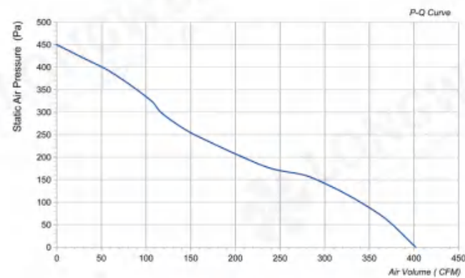
LWDE3G150-IS-05
