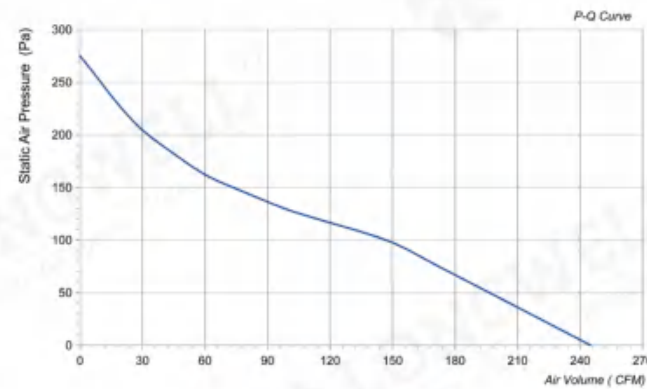
LWDE3G125-IS-01
