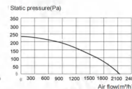
LWDA600S(T)-B03
