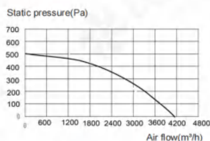
LWDA600S(T)-B05
