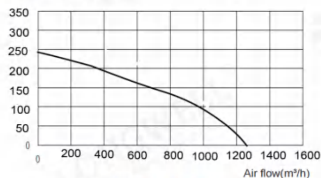
LWDA400S(T)-B01
