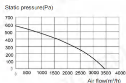
LWDA600S(T)-B04
