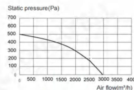
LWDA600S(T)-B01
