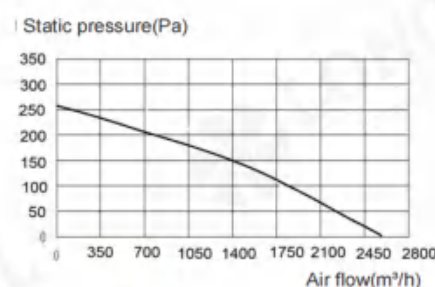
LWDA600S(T)-B06
