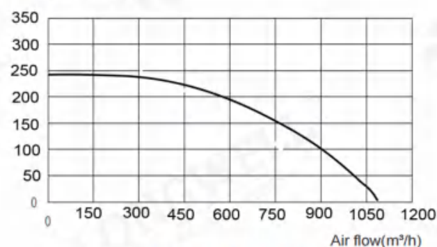
LWDA400S(T)-F01
